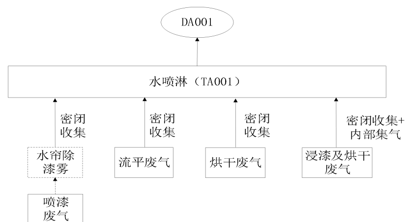
图 4-1 项目废气处理工艺流程图
