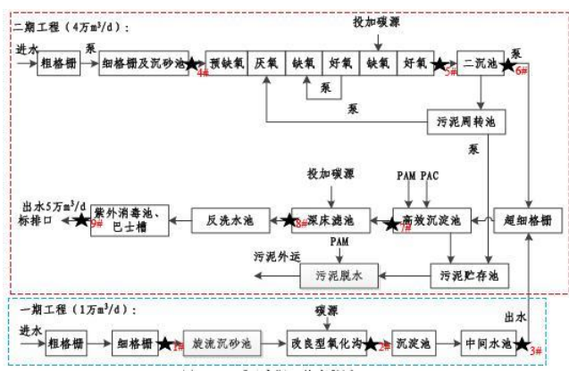
图 4-4 一二期工程污水处理工艺流程图
