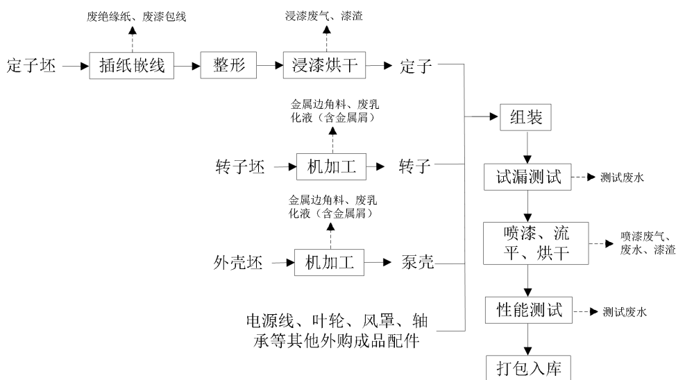
图 2-3 水泵生产工艺及产污环节示意图
