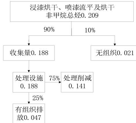
图 2-2 本项目涂料溶剂平衡图 单位 t/a
