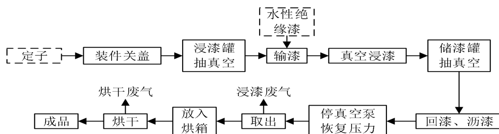
图 2-4 真空浸漆工艺流程图
