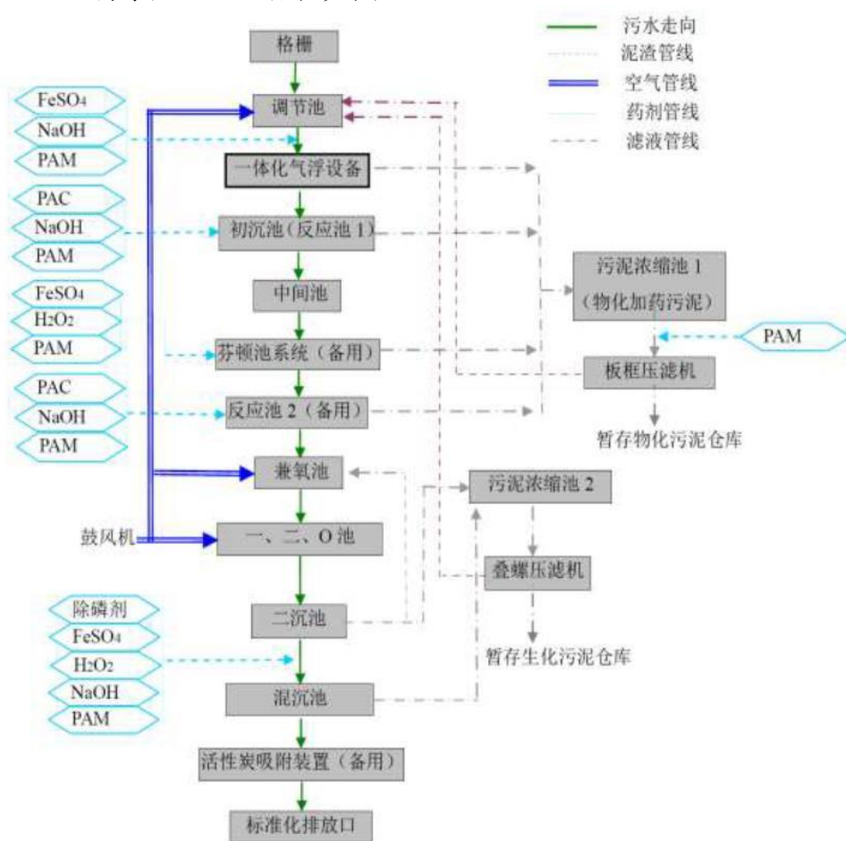
图 4-3 污水处理工艺流程图
